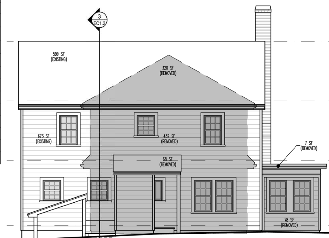
2 SCALE: 1/8" = 1'-0" WEST ELEVATION
